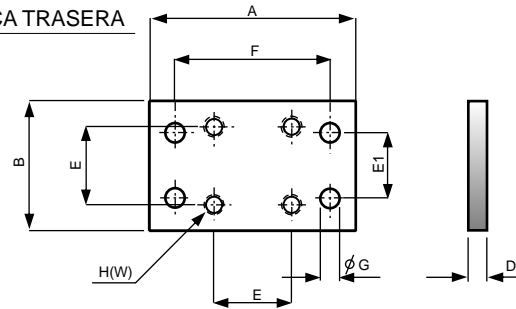
PLACA TRASERA
